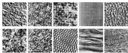
Fig. 4. Texture dataset 2
