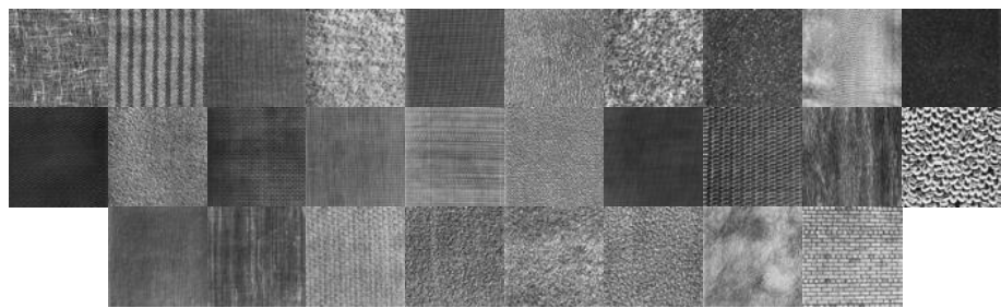
Fig. 3. Texture dataset 1
