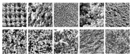
Fig. 5. Texture dataset 3
