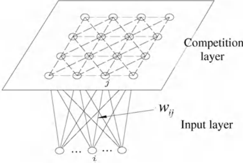
Fig. 1. SOM Network Structure
